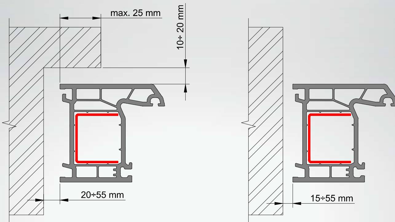
Рис. 4.1.1. Оконные блоки из ПВХ профилей белого цвета при размере стороны до 2000 мм.
