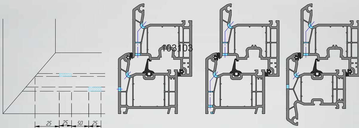
Рис. 3.2.2. Выполнение отвода воды на раме, створке и импосте
