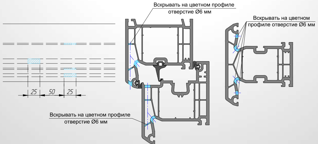
Рис. 3.2.1. Выполнение вентиляции на раме, створке и импосте
